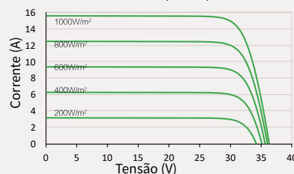
Potência-Tensão (450W)
