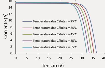
Corrente-Tensão (450W)
